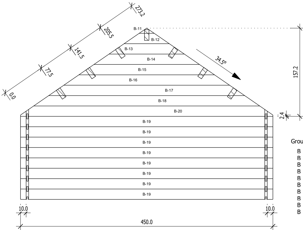
Ansicht von Innen Gegnes 8.0x19.0
