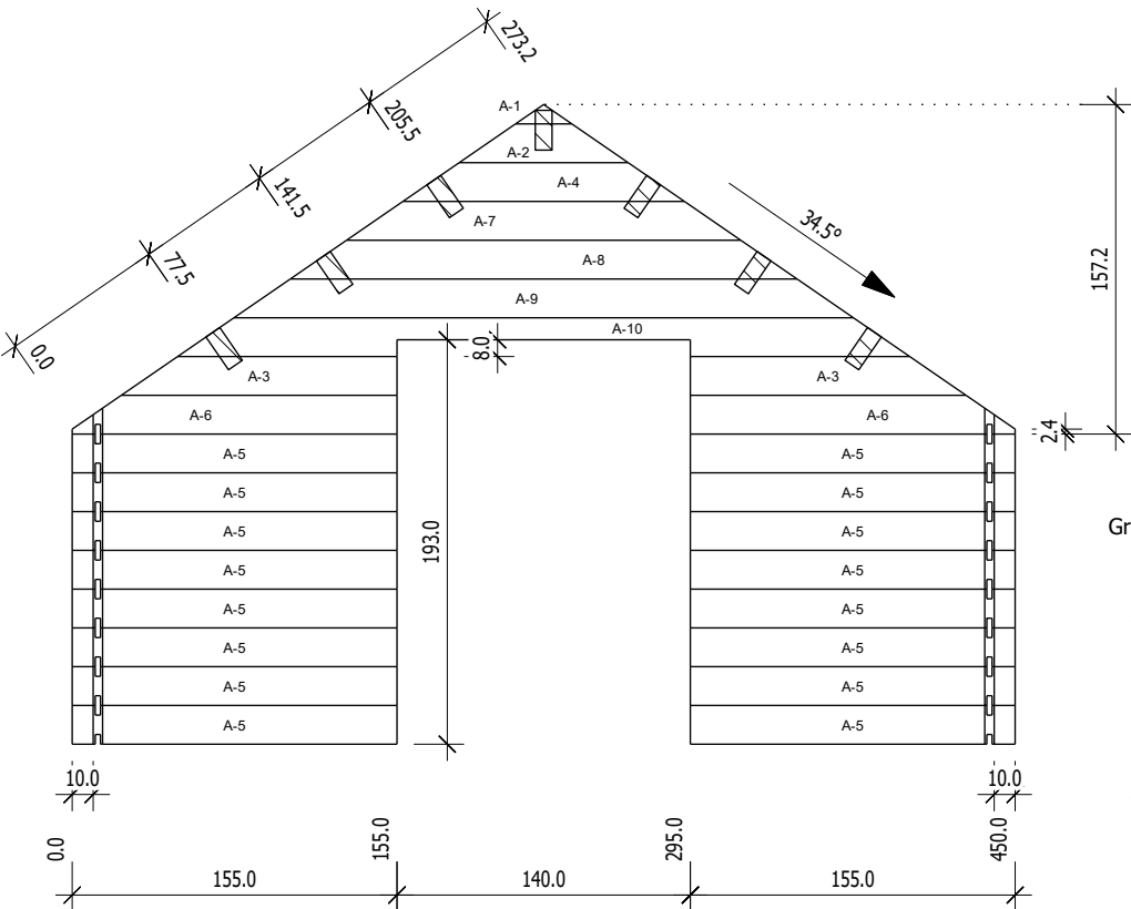
Ansicht von Aussen Gegnes 8.0x19.0
