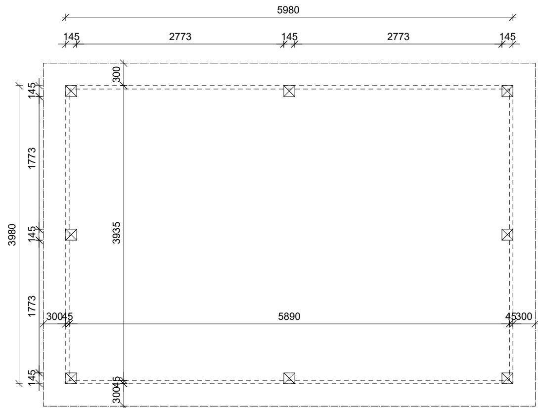
Platte grond
