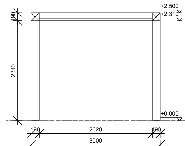
Verticale doorsnede
