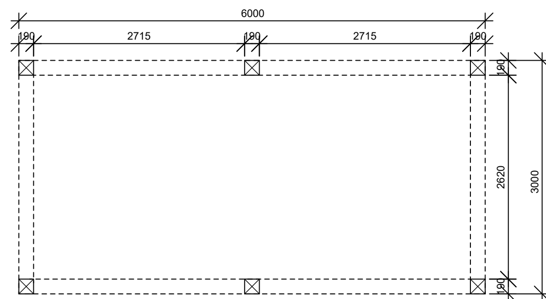
platte grond
