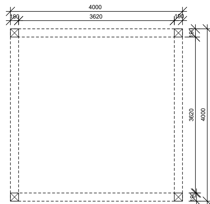
platte grond
