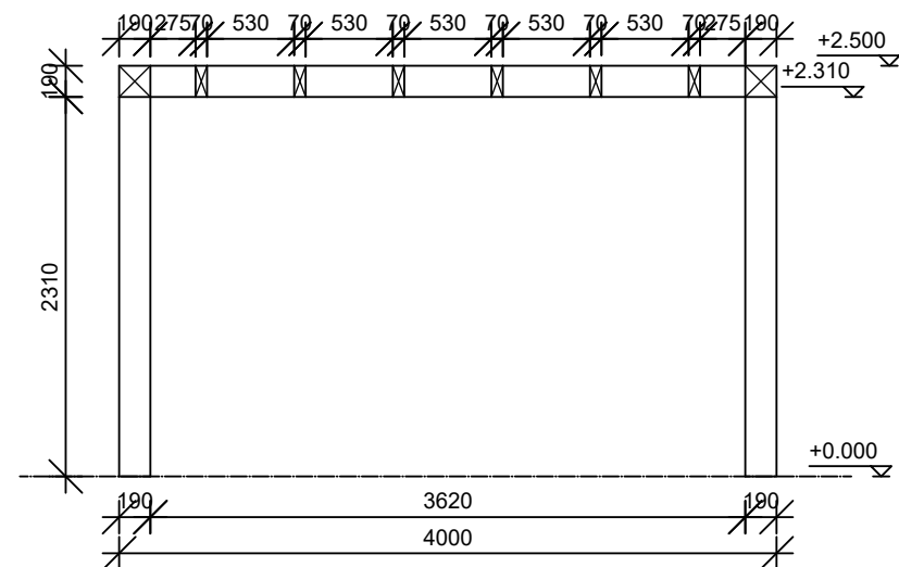
Horizontale doorsnede
