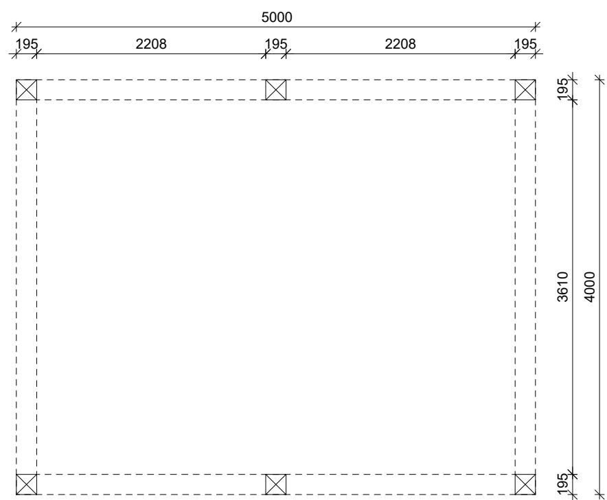
platte grond
