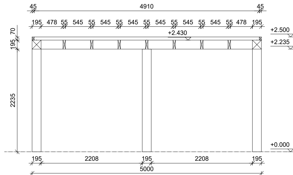
Horizontale doorsnede
