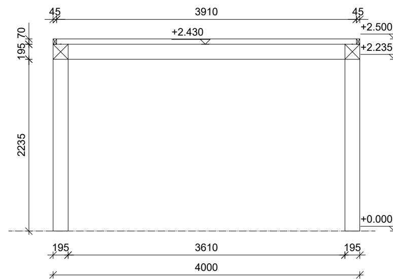
Verticale doorsnede
