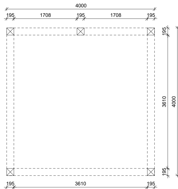
platte grond
