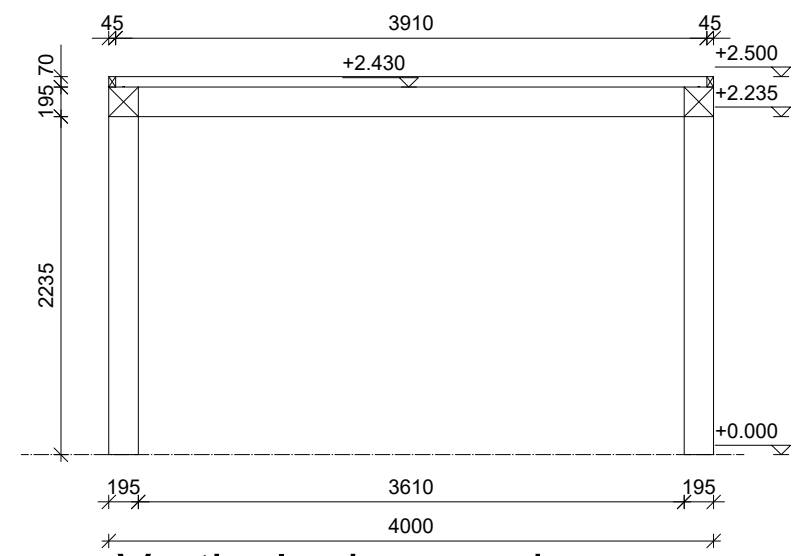
Verticale doorsnede
