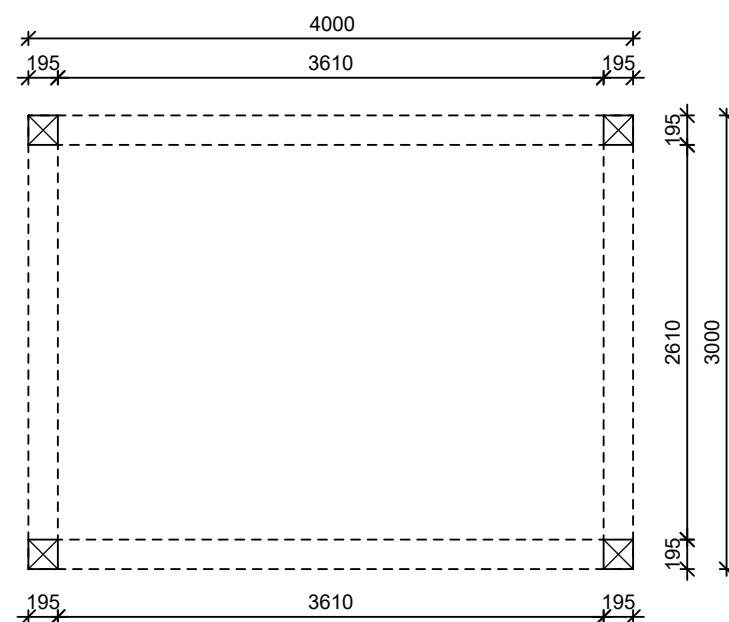
platte grond
