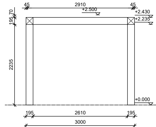
Verticale doorsnede
