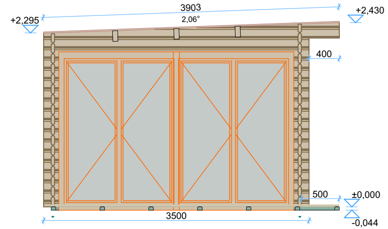
Right Elevation
