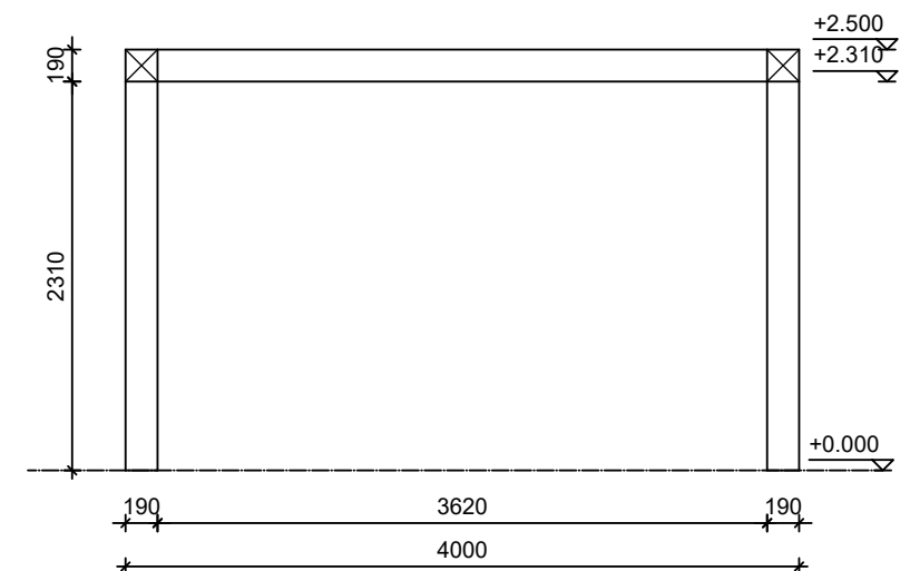
Verticale doorsnede
