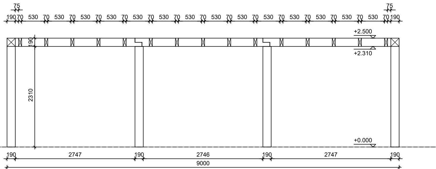
Horizontale doorsnede
