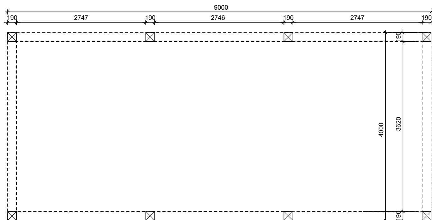
platte grond
