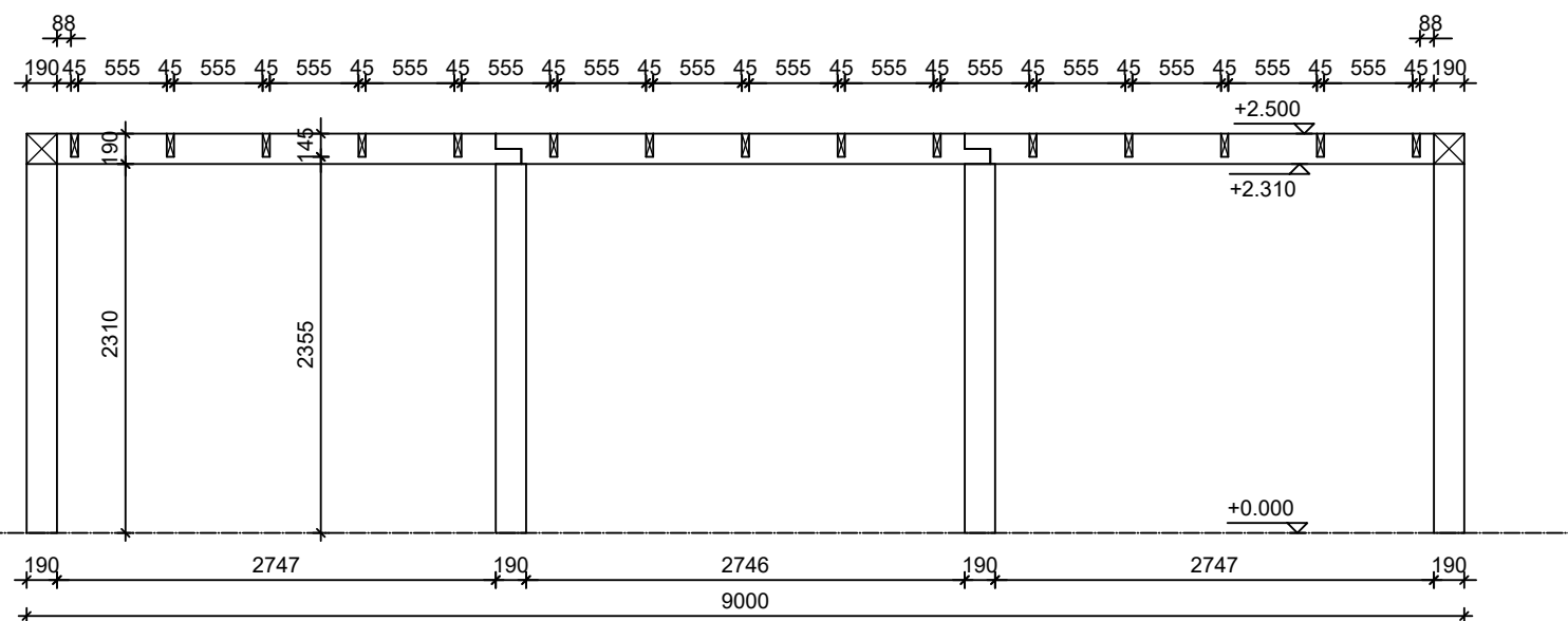
Horizontale doorsnede
