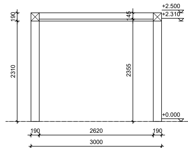
Verticale doorsnede
