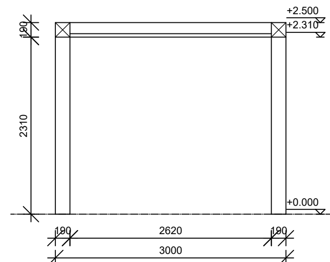
Verticale doorsnede
