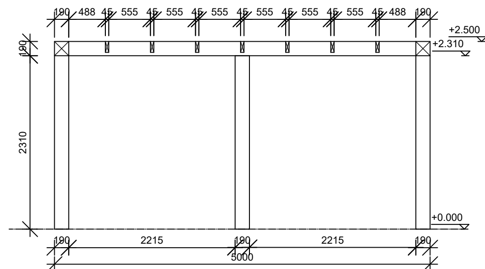
Horizontale doorsnede
