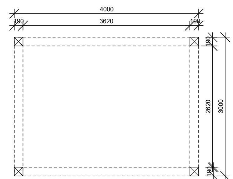
platte grond
