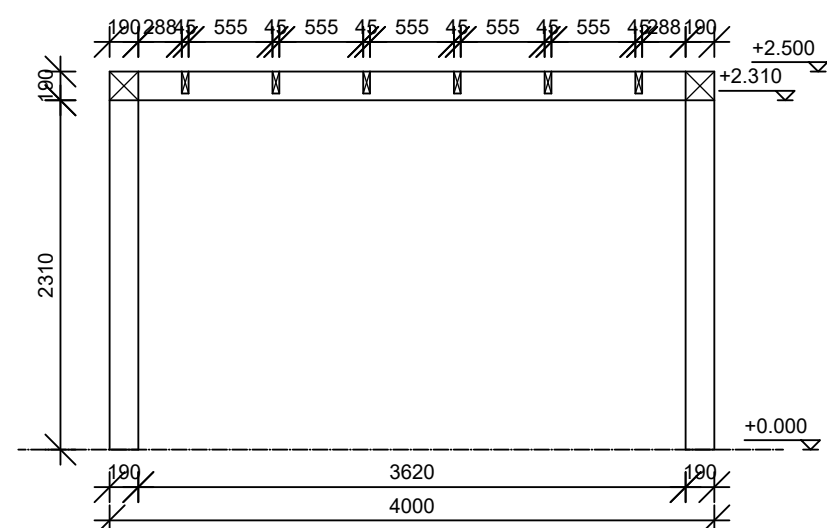
Horizontale doorsnede
