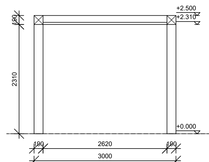
Verticale doorsnede
