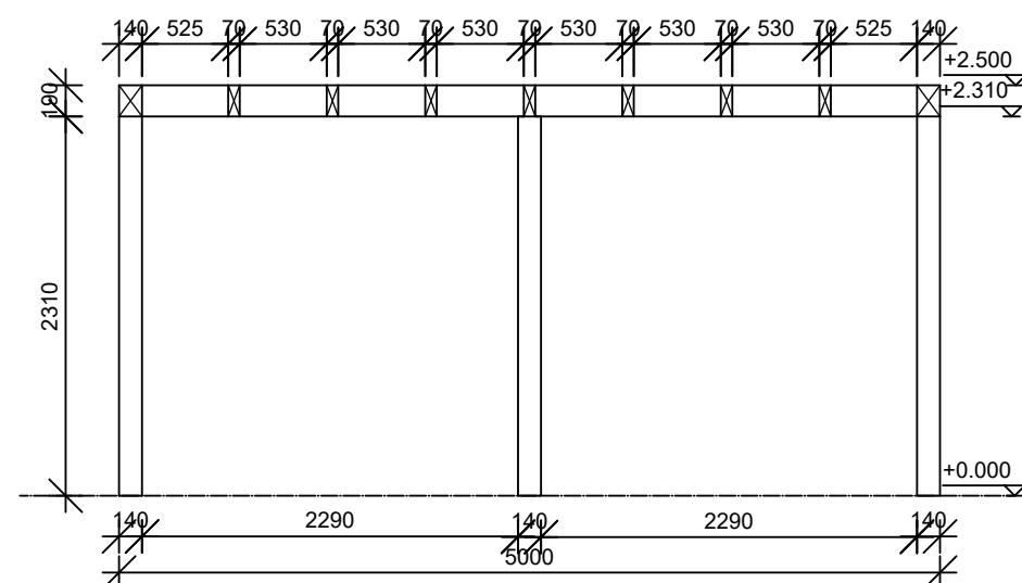
Horizontale doorsnede
