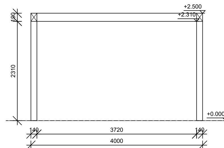
Verticale doorsnede
