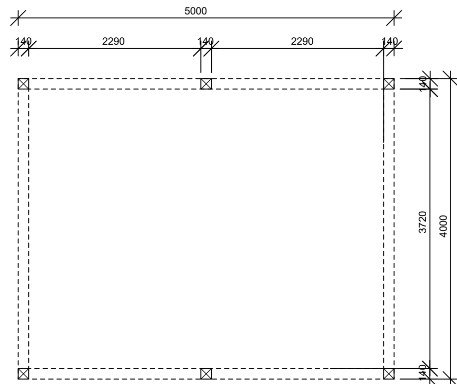
platte grond
