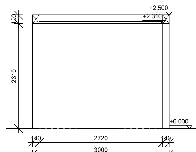
Verticale doorsnede
