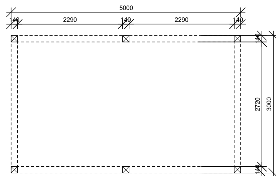
platte grond
