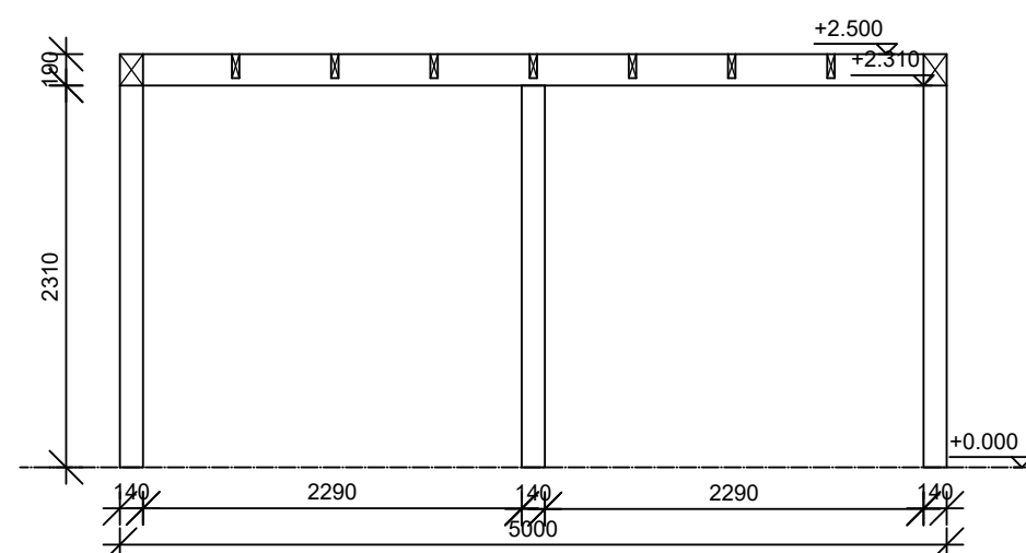
Horizontale doorsnede
