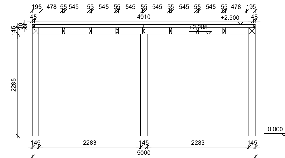
Horizontale doorsnede
