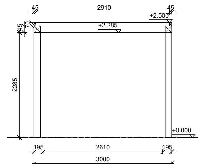
Verticale doorsnede
