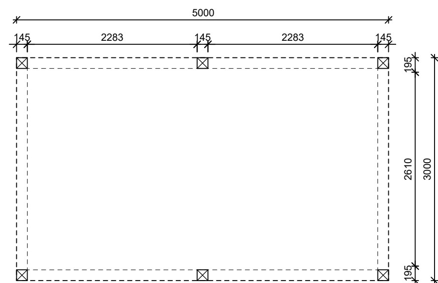
platte grond
