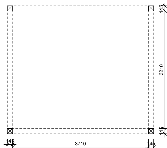
platte grond
