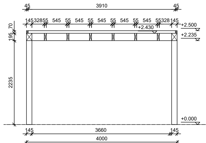
Horizontale doorsnede
