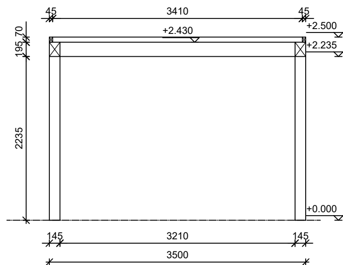
Verticale doorsnede
