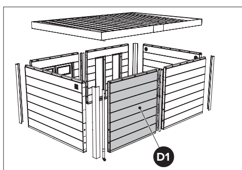
D1 Paroi / Wand / Wall / Wand
