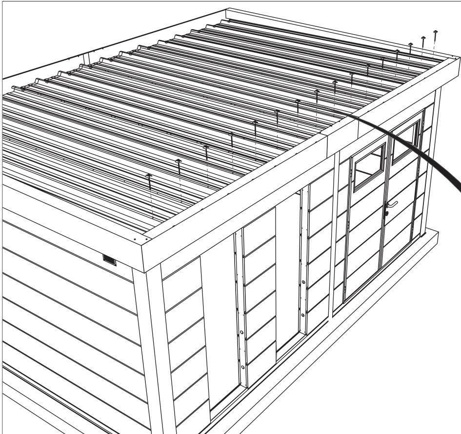
Toit / Dak / Roof / Dach
