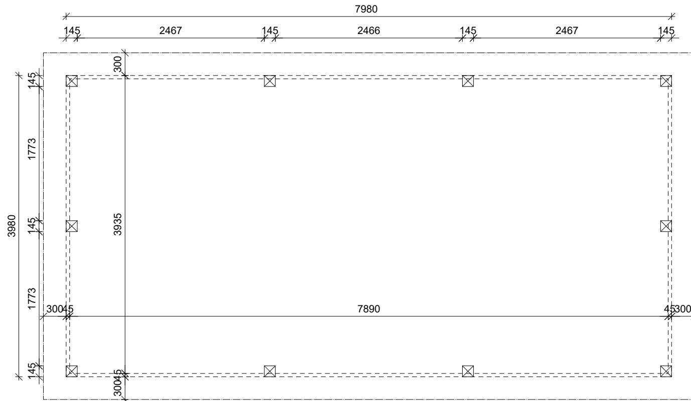
Platte grond
