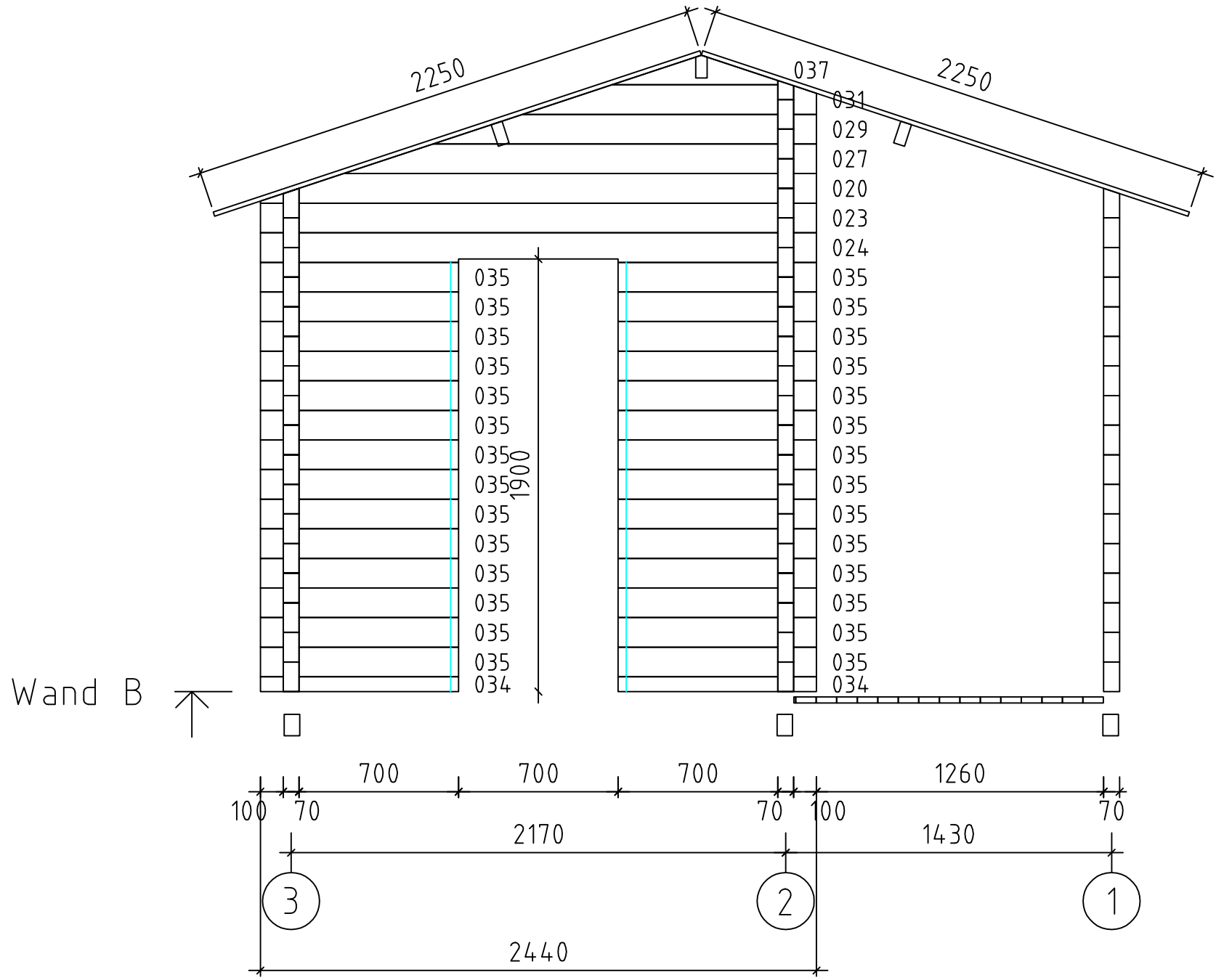
Aussensauna 3940 / 70 / 13
