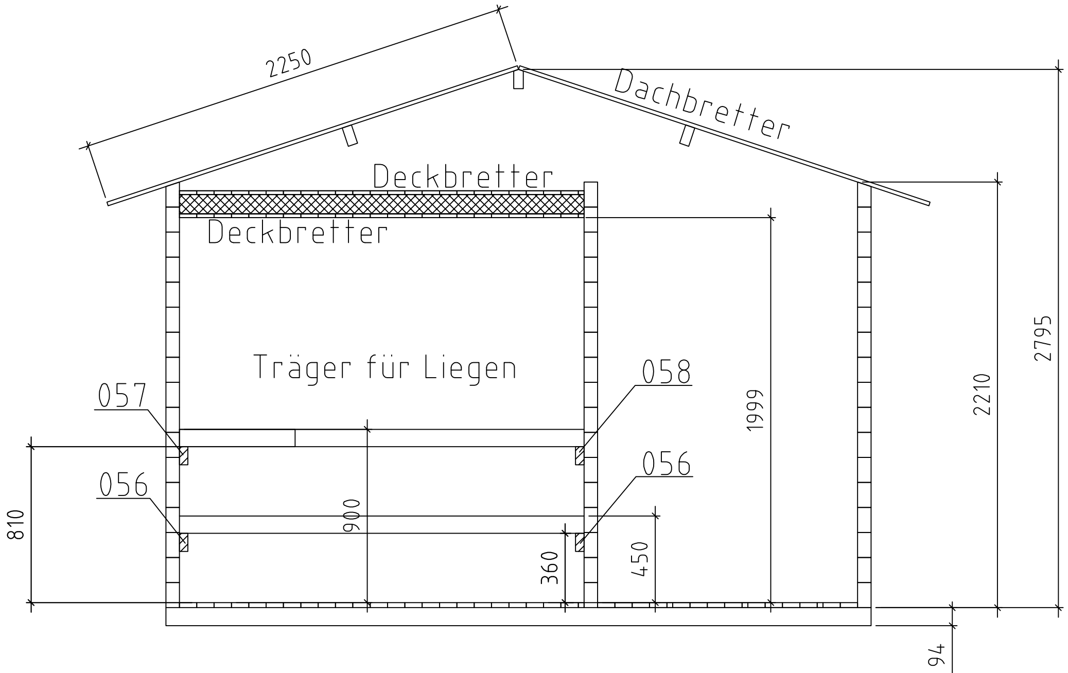
Aussensauna 3940 / 70 / 13
